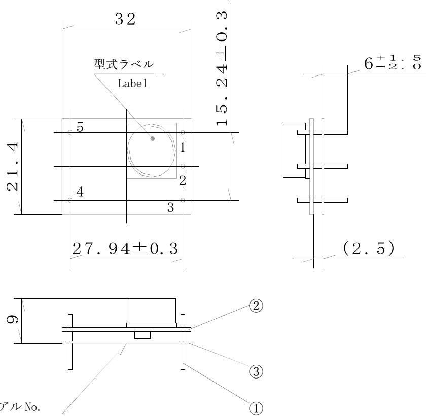
端子接続図 Pin Connection
