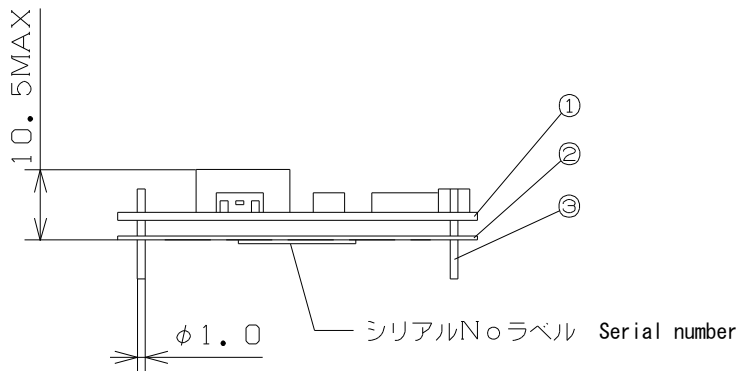
端子接続図 Pin Connection
