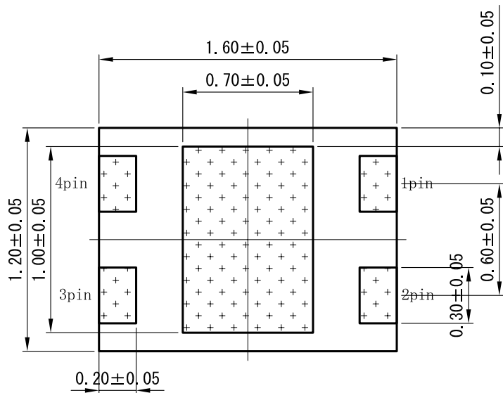
実装面
