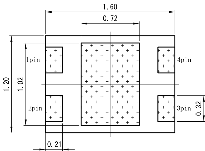
インナーリード部図
